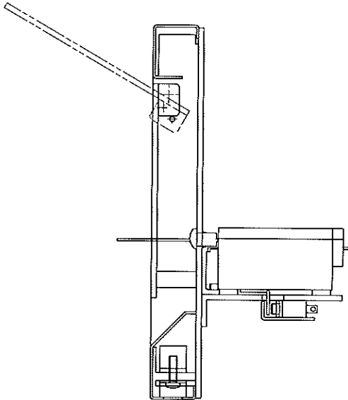
A-A断面
